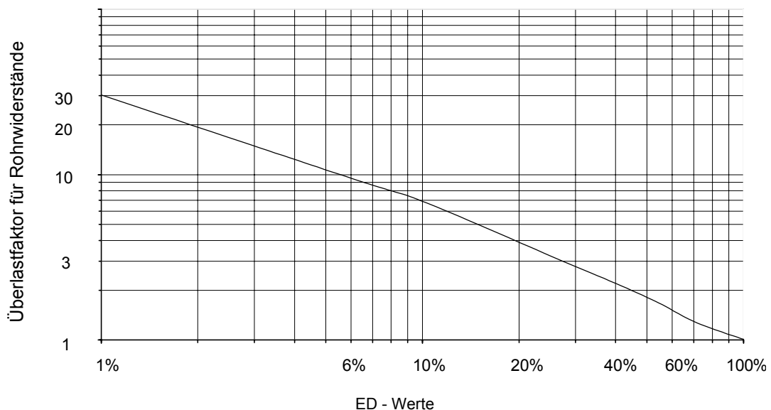
Überlastfaktor in Abhängigkeit der Einschaltdauer (Spieldauer 120s)
