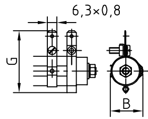
FZB / FUB 75 x 24 ST - FZB / FUB 300 x 45 ST mit Steckschellen / with fast-on clips mit 1 Abgreifschelle / with 1 adjustable clip FZB / FUB 75 x 24 S2T - FZB / FUB 300 x 45 S2T mit 2 Abgreifschellen / with 2 adjustable clips FZB / FUB 75 x 24 SnT - FZB / FUB 300 x 45 SnT mit n Abgreifschellen / with n adjustable clips
