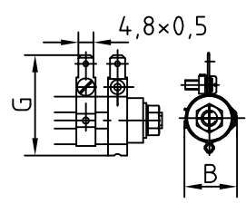
FZB / FUB 50 x 16 AE - FZB / FUB 100 x 16 AE mit Steckschellen / with fast-on clips mit 1 Abgreifschelle / with 1 adjustable clip FZB / FUB 50 x 16 A2E - FZB / FUB 100 x 16 A2E mit 2 Abgreifschellen / with 2 adjustable clips FZB / FUB 50 x 16 AnE - FZB / FUB 100 x 16 AnE mit n Abgreifschellen / with n adjustable clips
