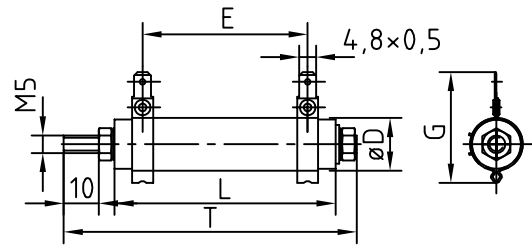
FZB / FUB 50 x 16 A - FZB / FUB 100 x 16 A mit Steckschellen / with fast-on clips ohne Abgreifschelle / without adjustable clip
