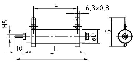
FZB / FUB 75 x 24 S - FZB / FUB 300 x 45 S mit Steckschellen / with fast-on clips ohne Abgreifschelle / without adjustable clip
